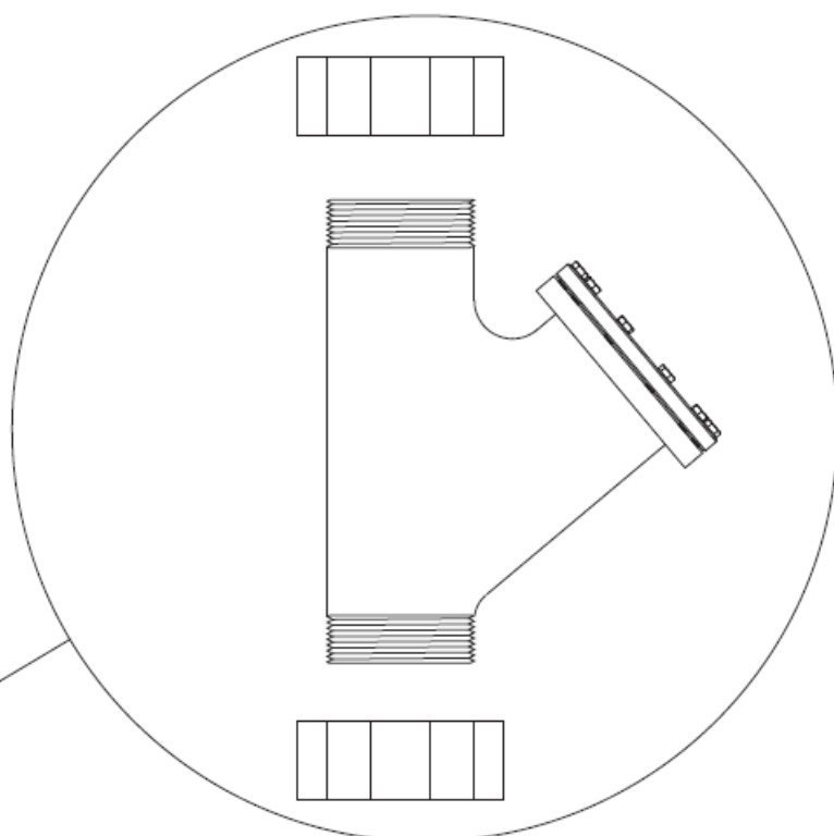
FILTRO Y
